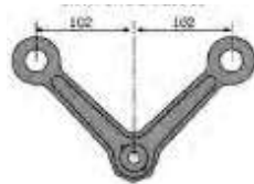
Sujeción de 2 brazos a 90°
